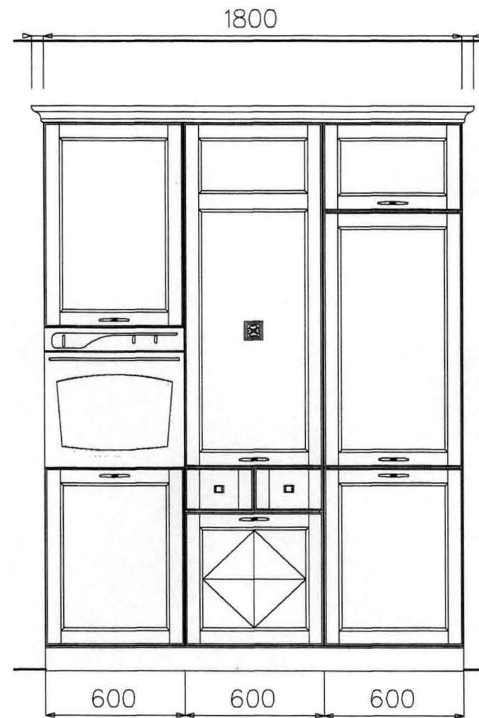
Prospetto B
