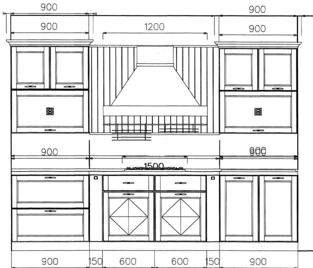
Prospetto A
